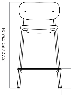
W: 49,4 cm / 19,45"
